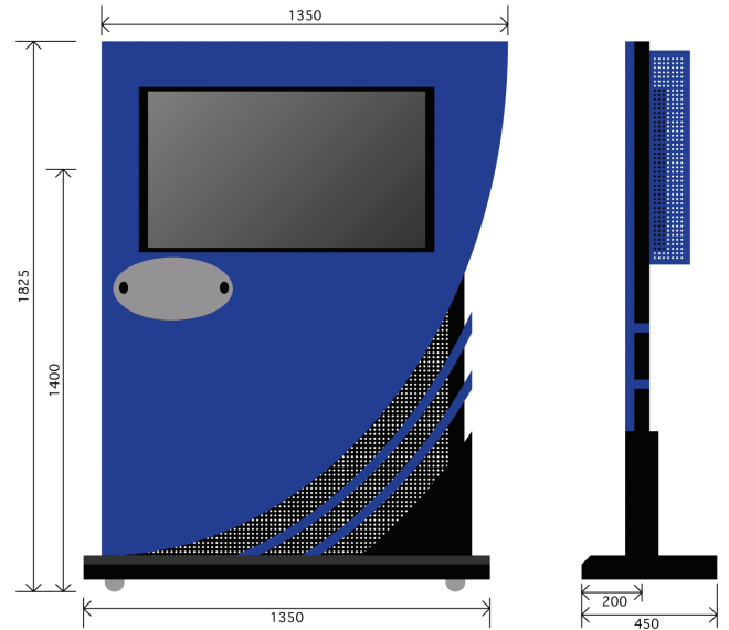
横型 (W1350×H1825×D450)
