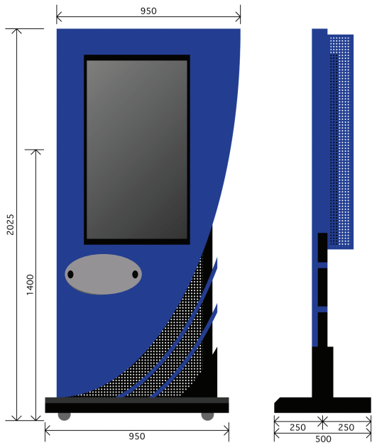
縦型 (W950×H2025×D500)
